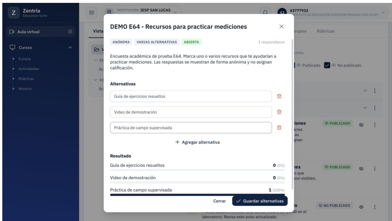
Figura 10. Contraste desde docente: mismos conteos y resultado sin nombres después de recargar.
